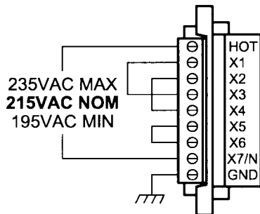
215VAC HOOKUP
