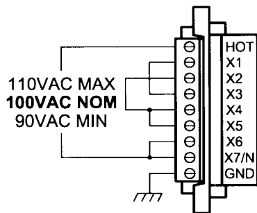
100VAC HOOKUP
